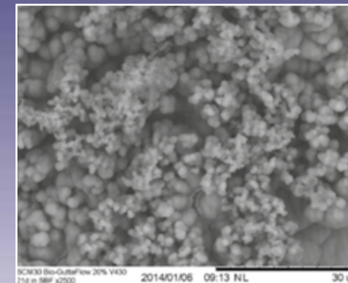
2500 x aumentos de los cristales de hidroxiapatita en la superficie de GuttaFlow bioseal bajo microscopio electrónico de barrido
